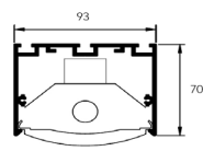
Rejilla parabólica
