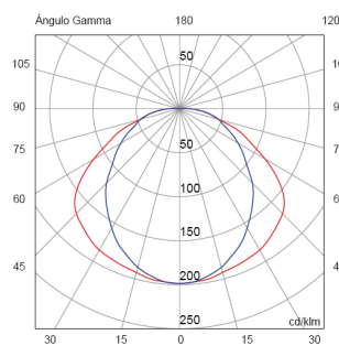
reflector simetrico lamas blancas
