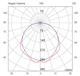
reflector simétrico brillo
