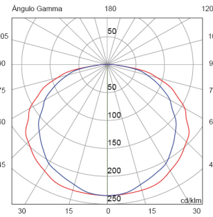
reflector simétrico blanco
