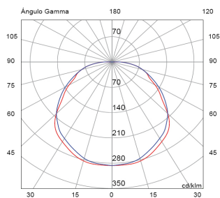
sin reflector
