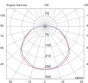
reflector y rejilla lamas blancas
