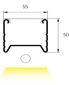
sin reflector
