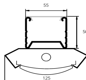
reflector y rejilla lamas curvas
