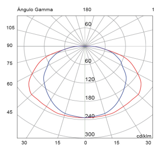
reflector simétrico blanco
