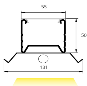
reflector simétrico
